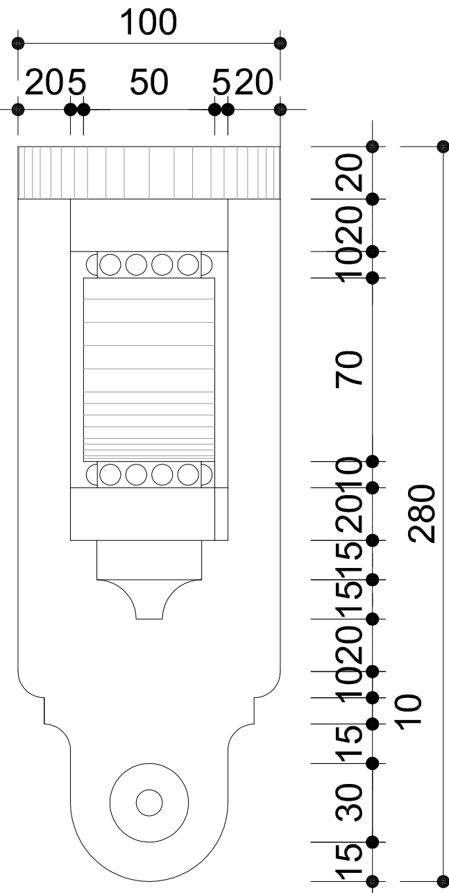
Vue frontale
