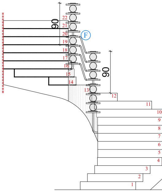
Détail F
