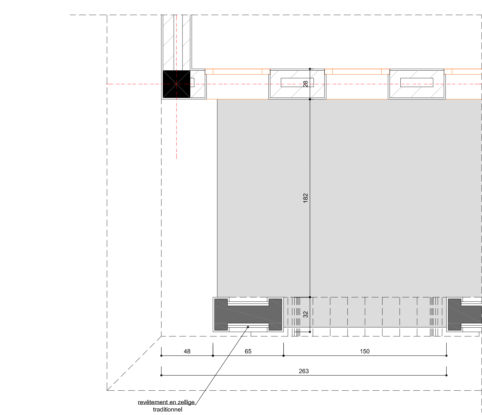
Plan Galerie Administration
