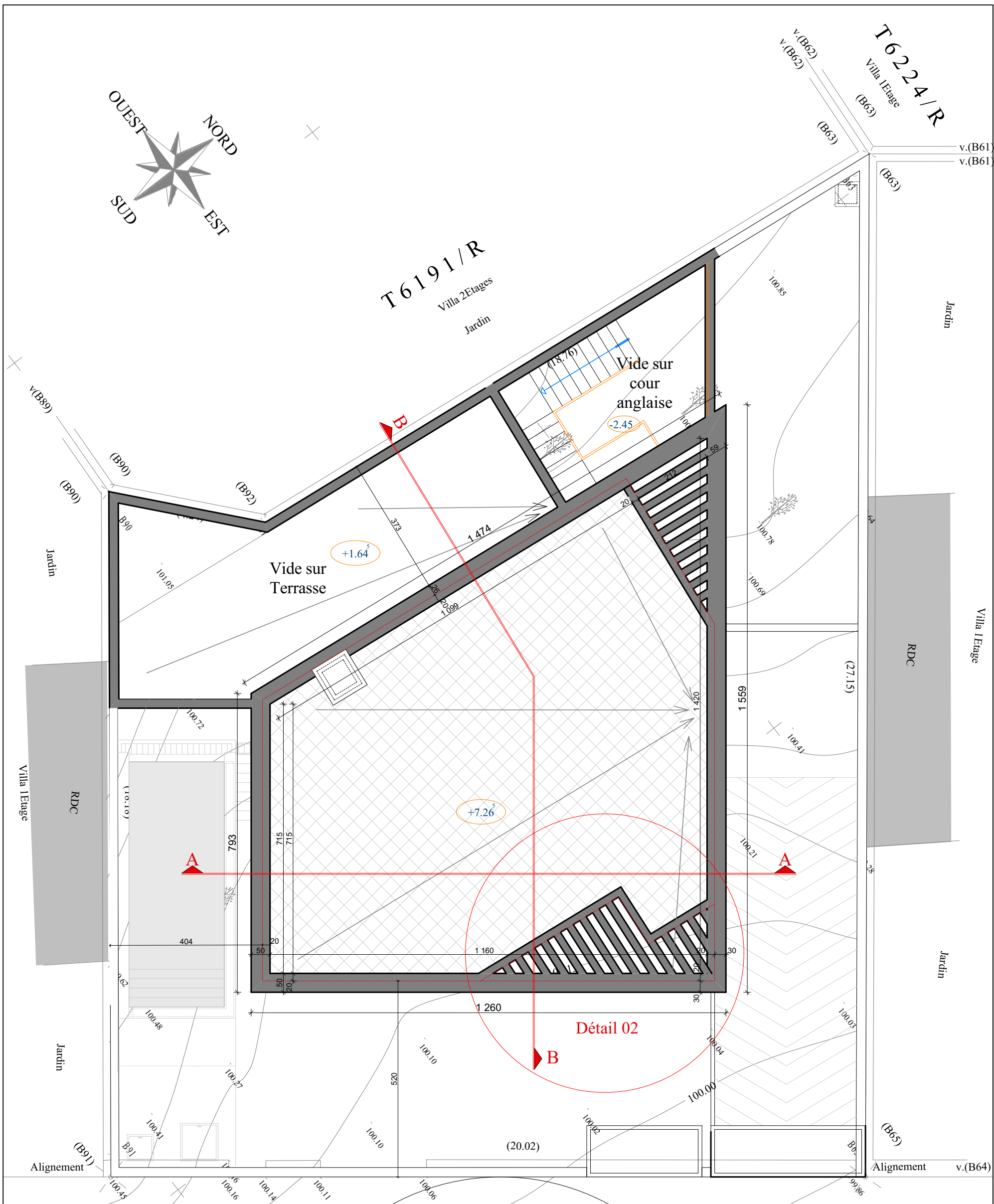
PLAN MASSE-TERRASSE
