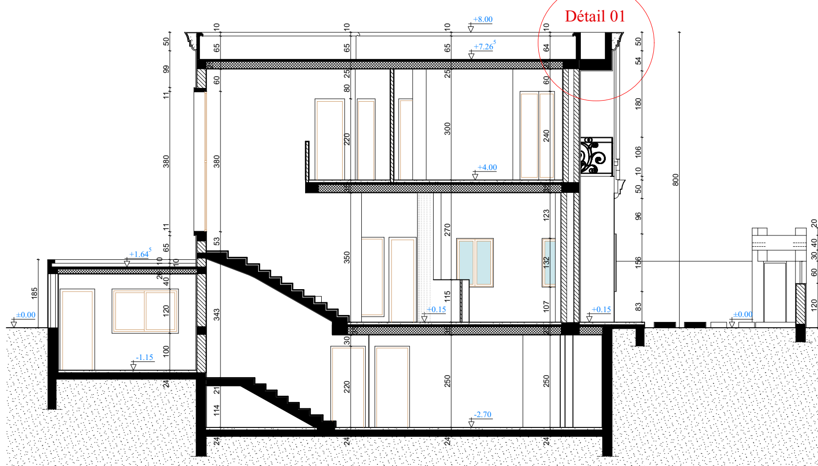
COUPE B-B
