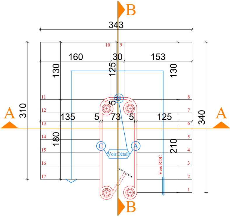
Plan escalier Sous Sol
