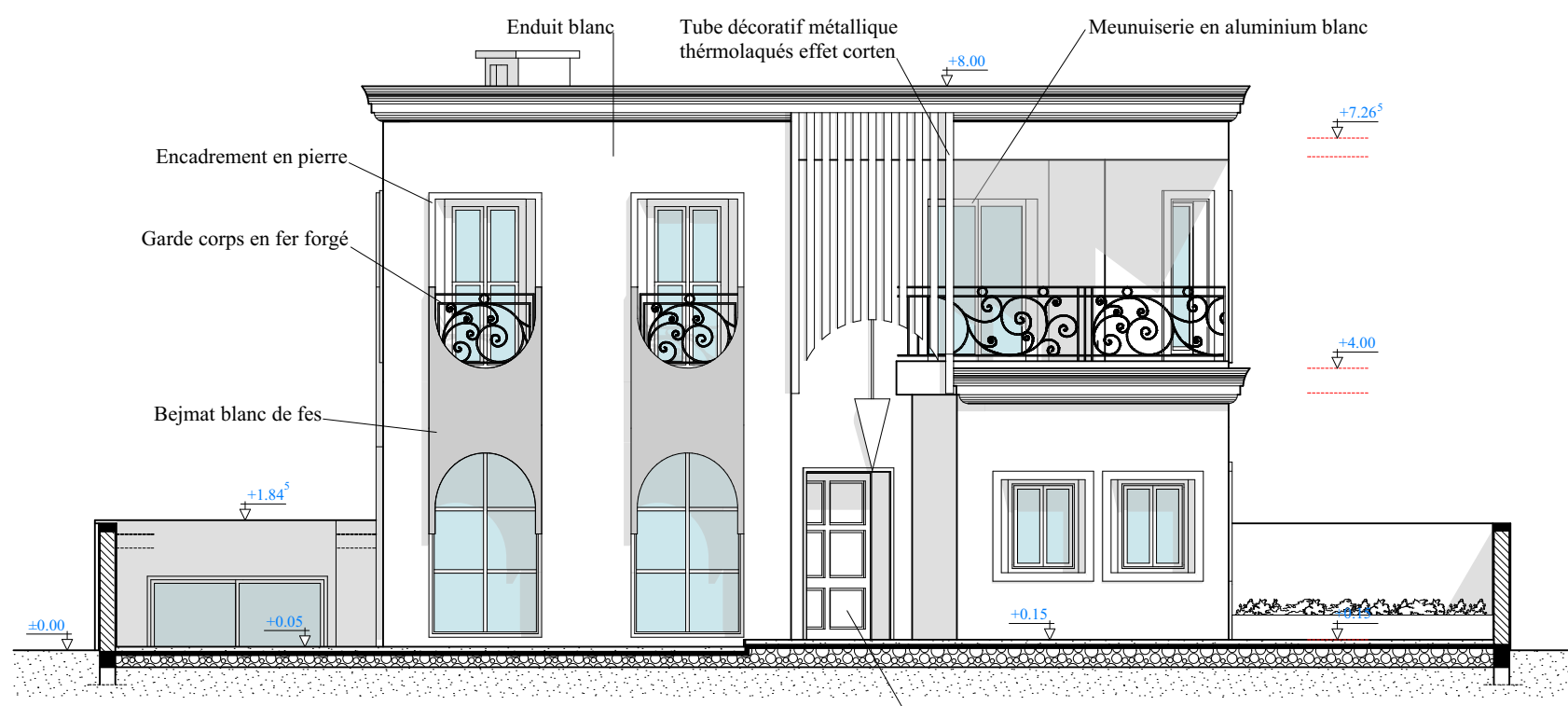
FACADE PRINCIPALE
