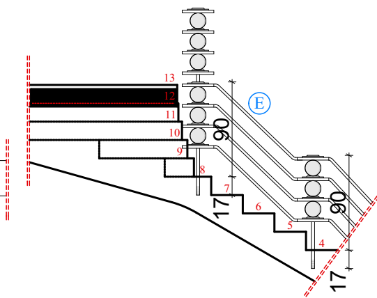
Détail E
