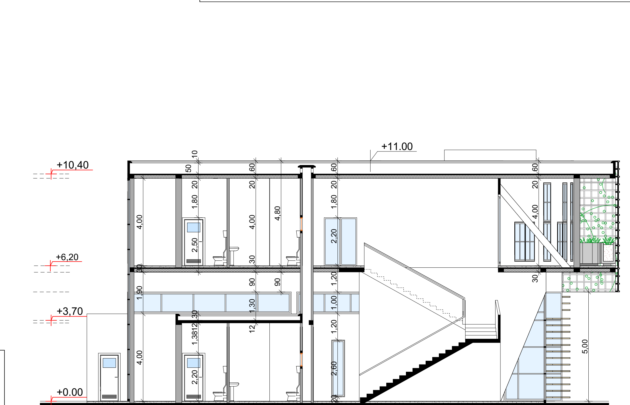
Coupe B-B
