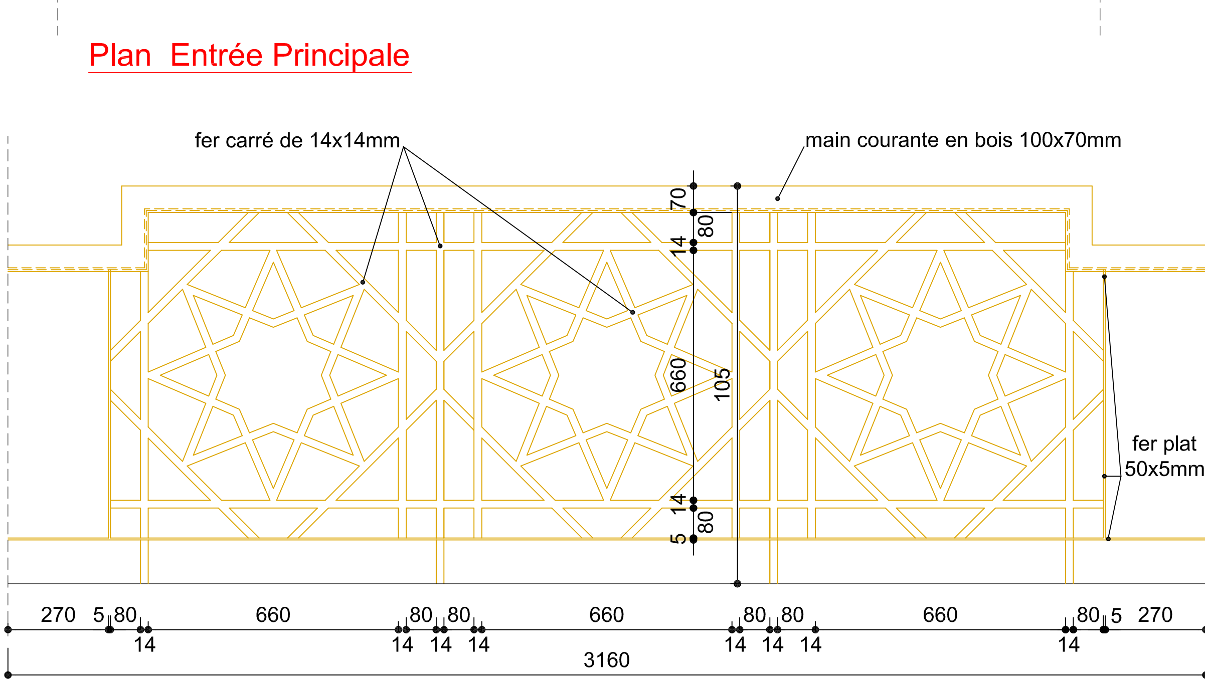
Détail Garde Corps
