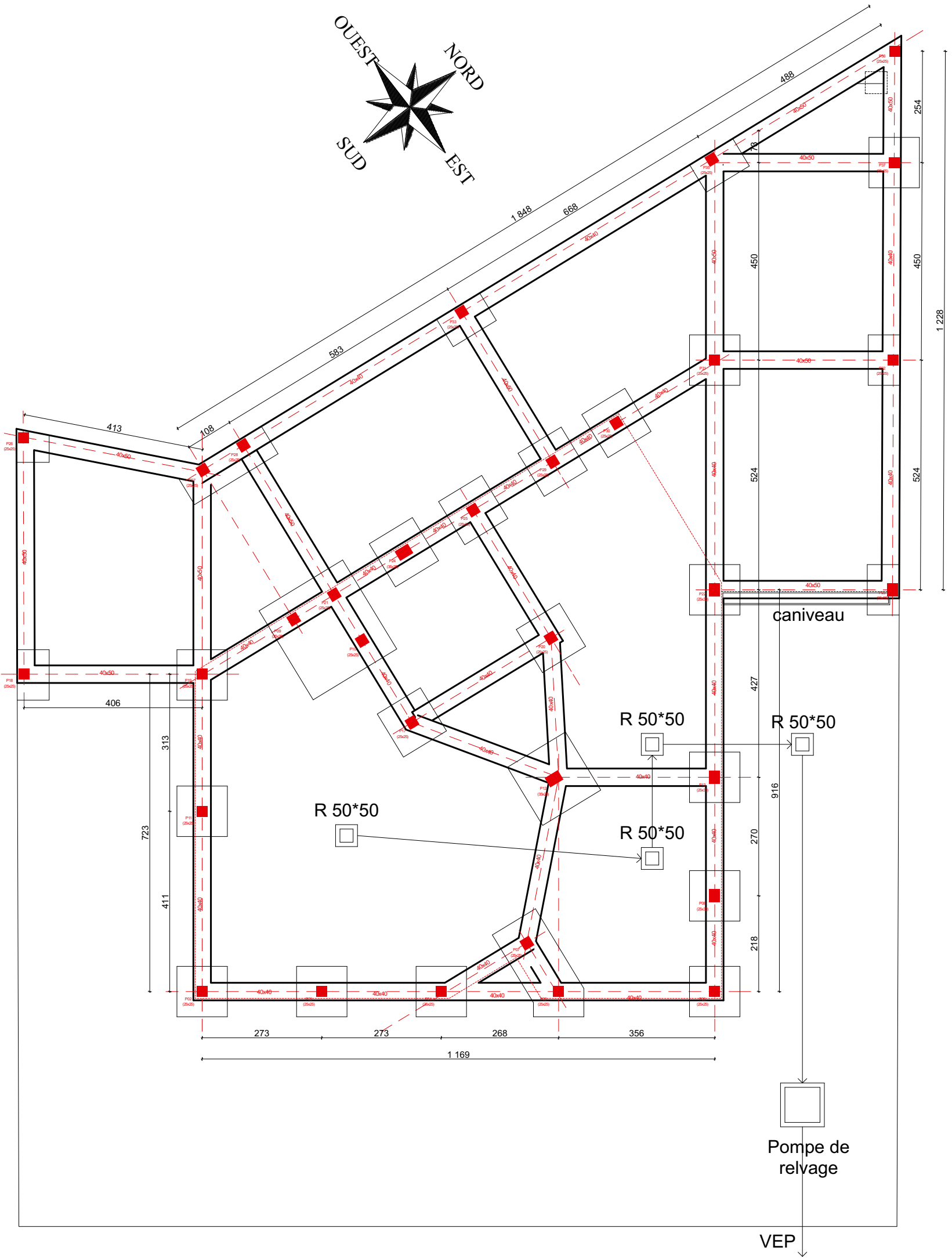
FONDATION
