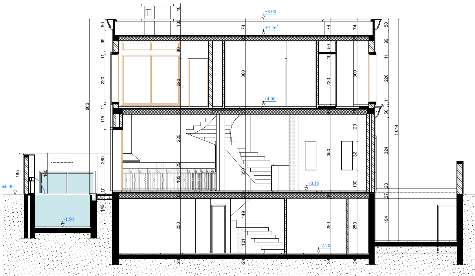
COUPE A-A
