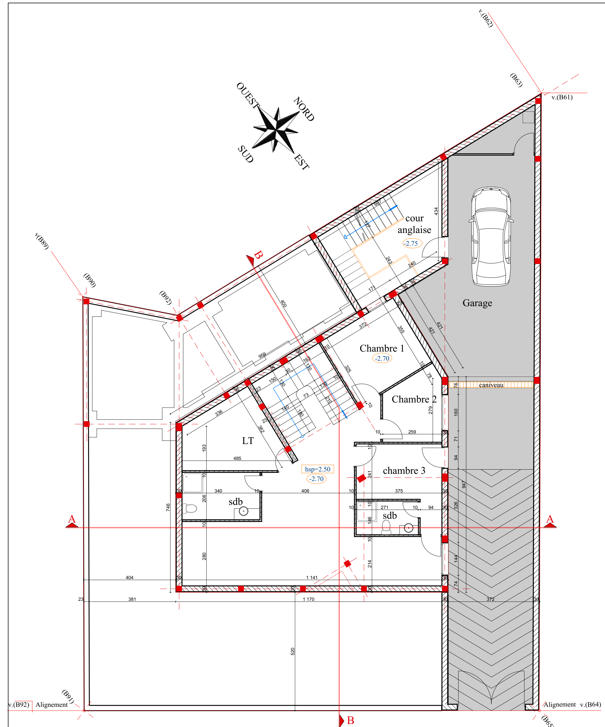
PLAN SOUS SOL
