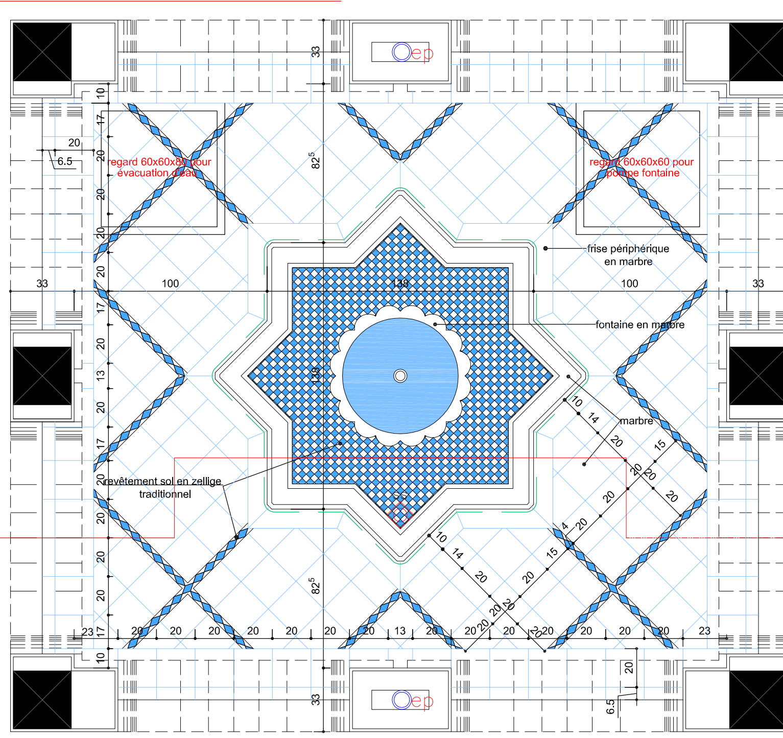
Plan détail C-C sur fontaine
