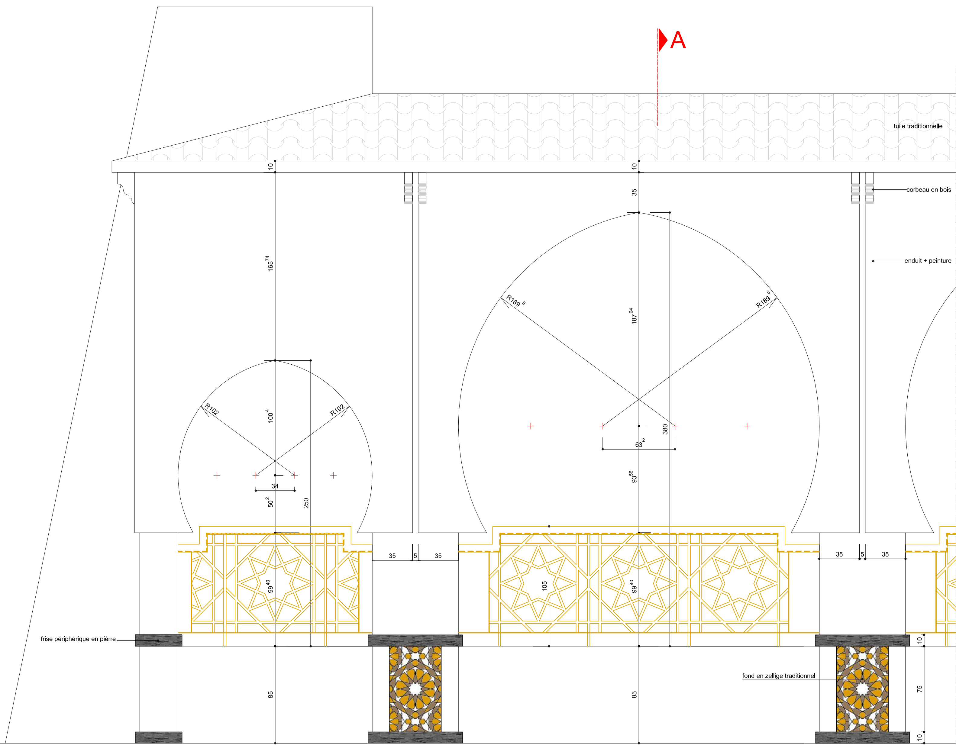
Elévation
