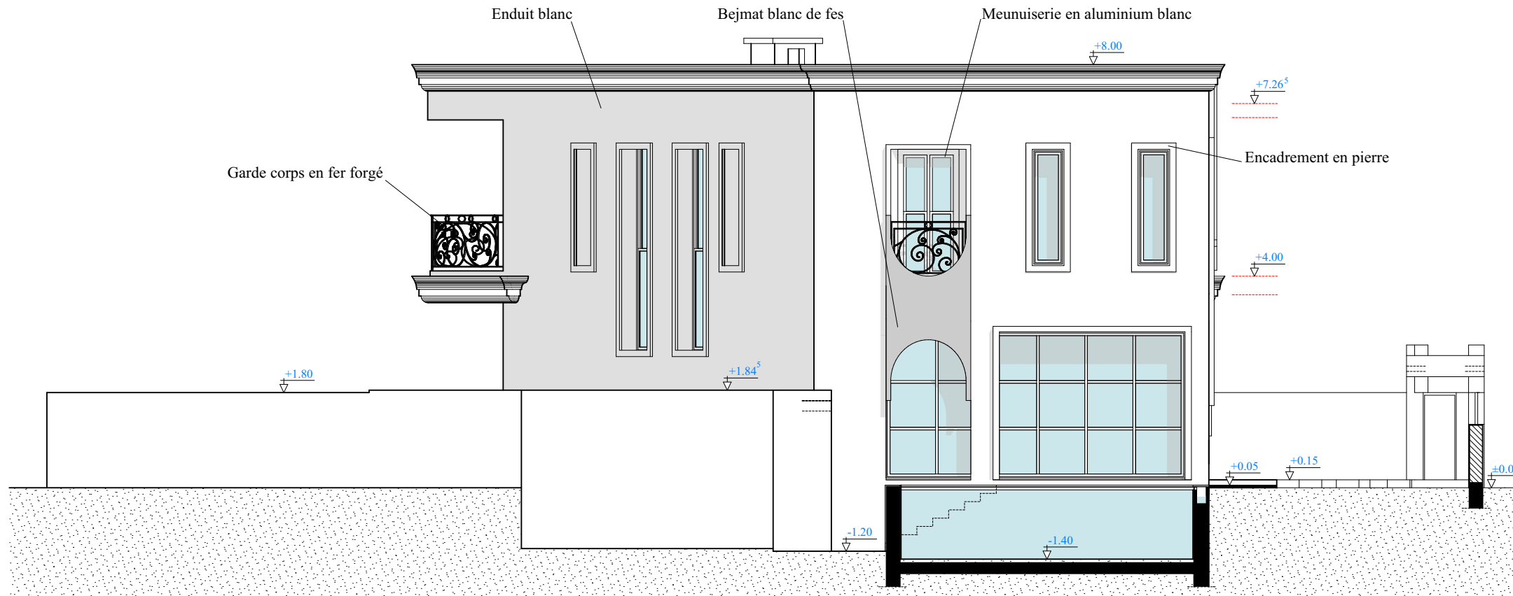
FACADE GAUCHE
