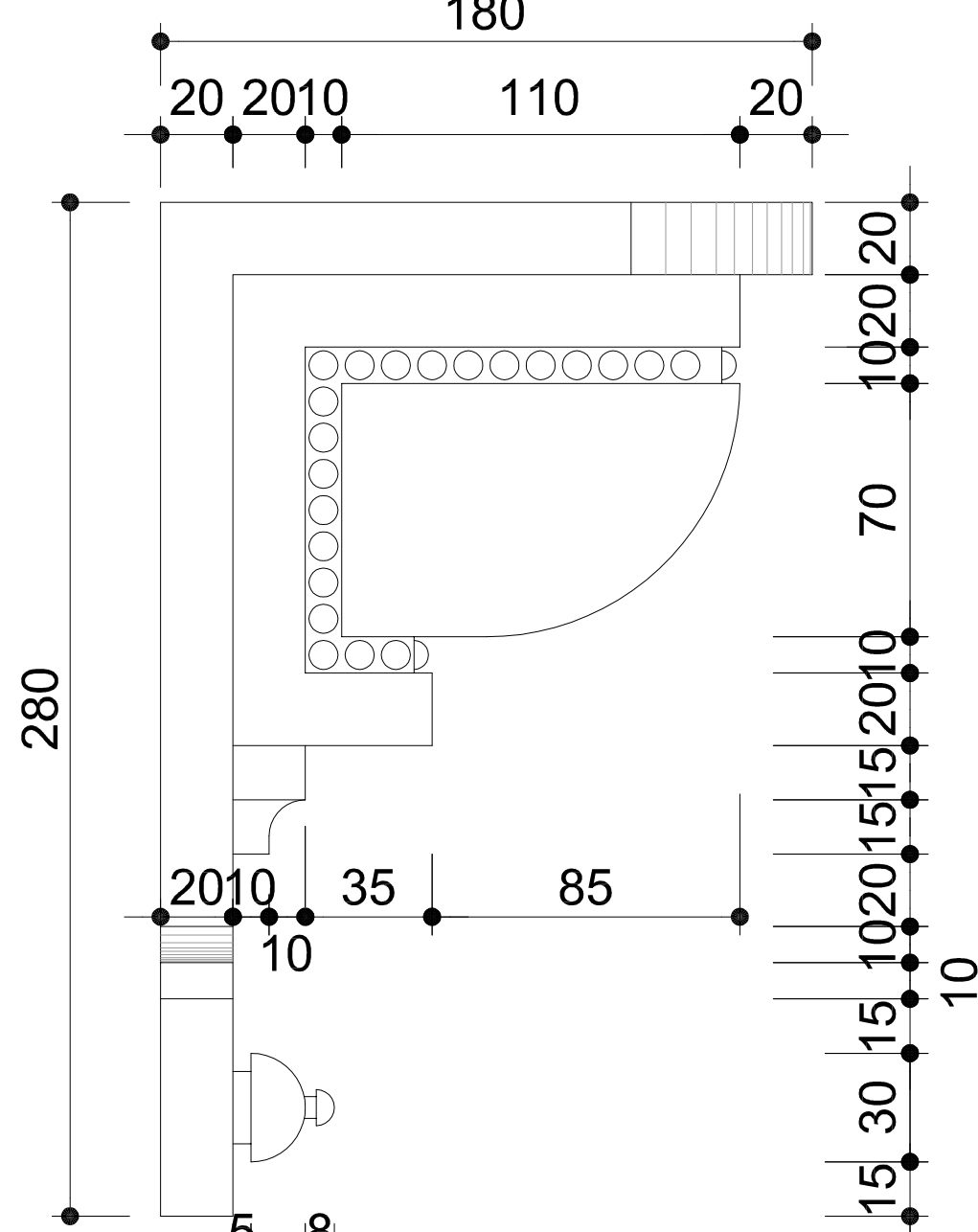
Vue de profil de la console
