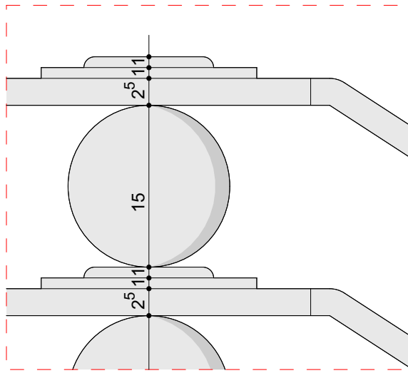
Détail 02
