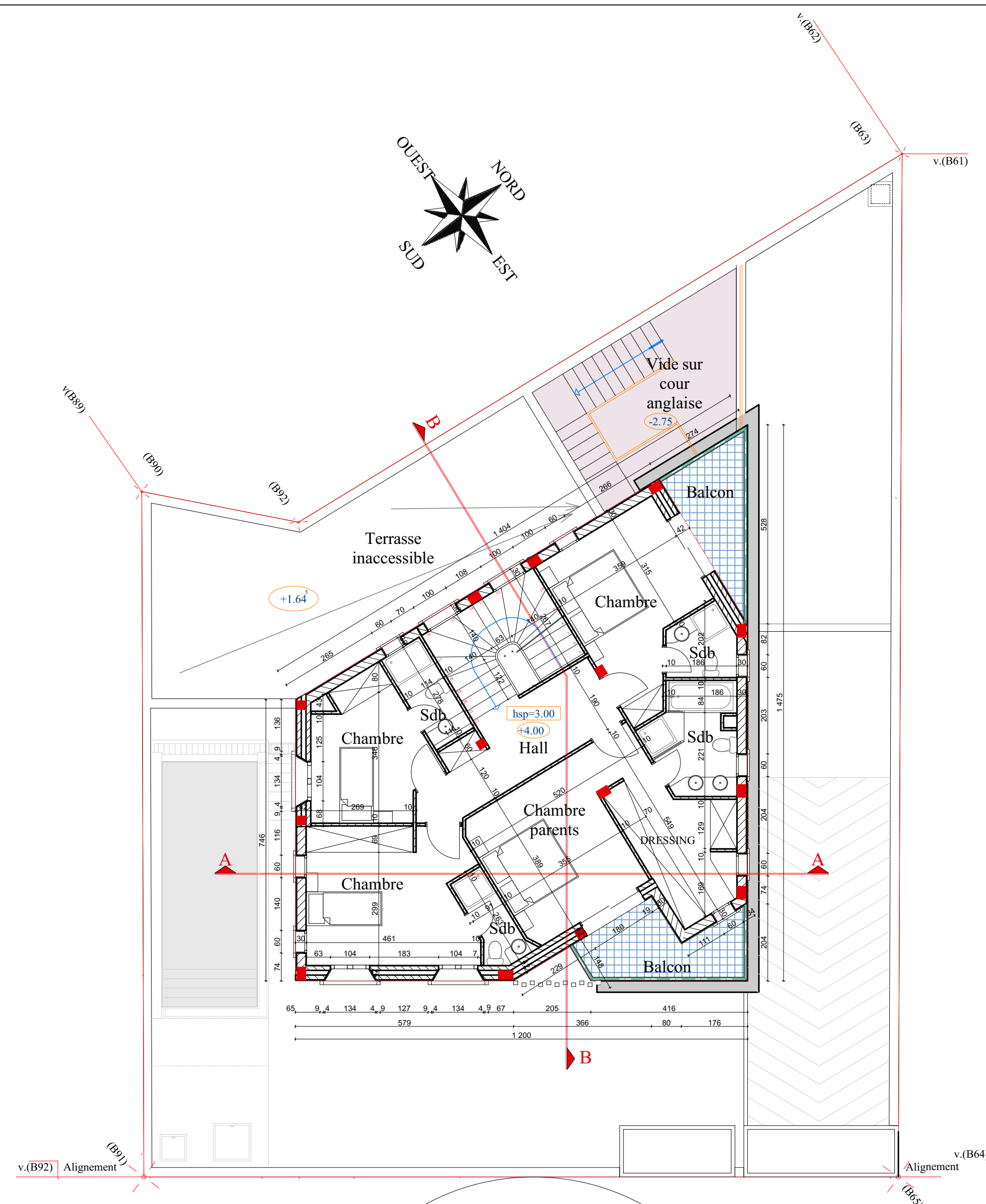
PLAN 1er ETAGE
