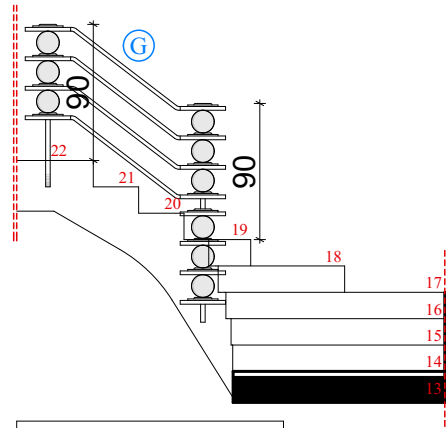
Détail G
