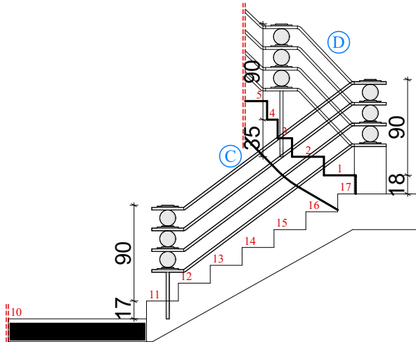
Détail C et D
