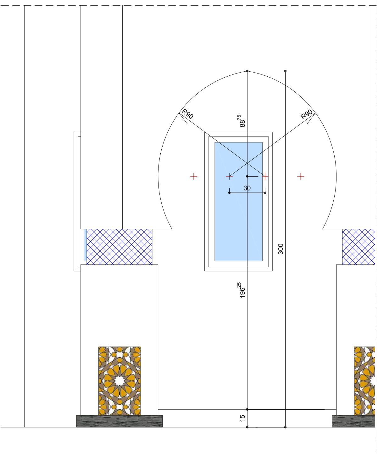
Elévation Galerie Administration
