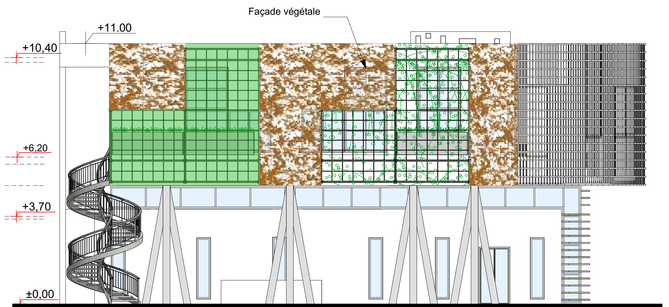
Façade Ouest
