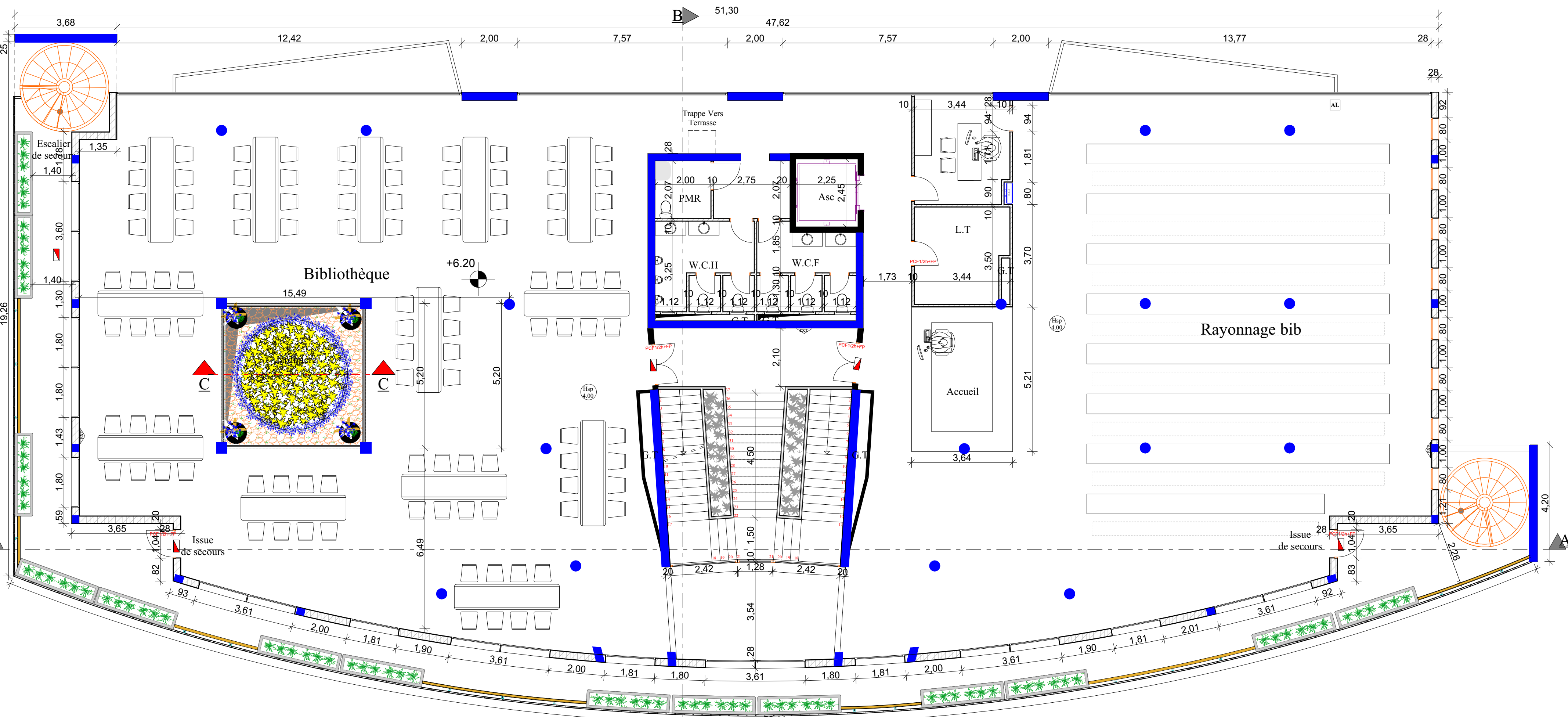
Etage
