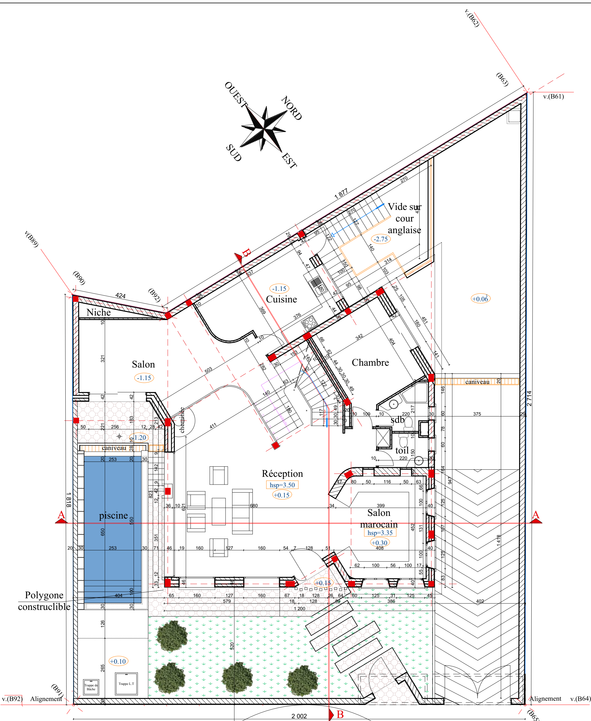
PLAN REZ DE CHAUSSEE
